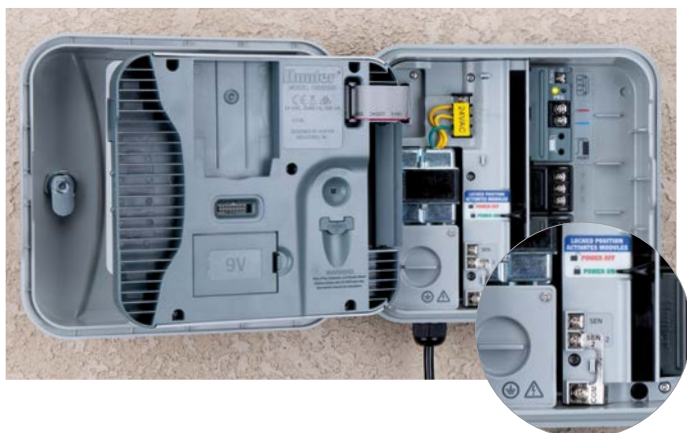
P2C-400 STEUERGERÄT MIT 2 SENSOREINGÄNGEN
