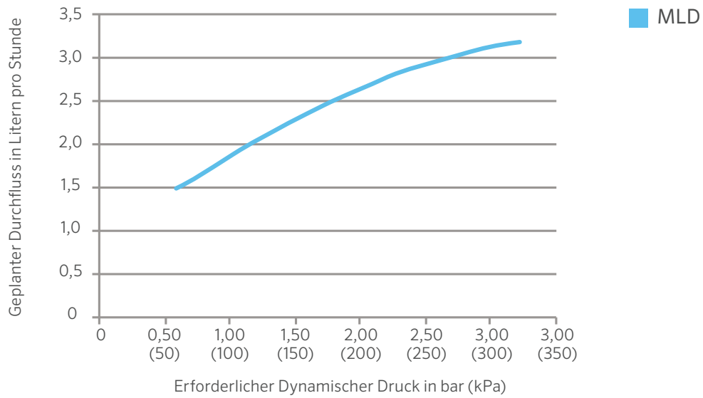
MLD FLUSS-TABELLE
